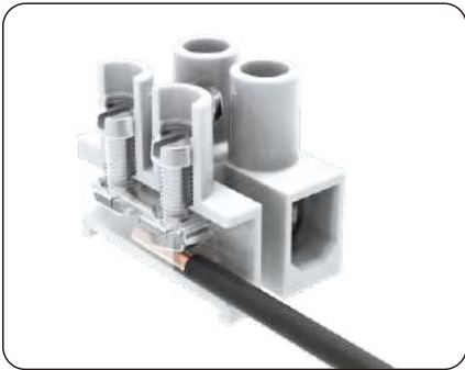
护线弹片设计 保护导线免受损伤
