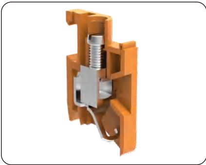
螺钉连接 提线框或垫片式螺钉连接稳定可靠
