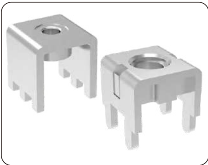
后制程铆螺母/一体化成型螺母 多种螺母制程工艺保证扭力数倍于标准
